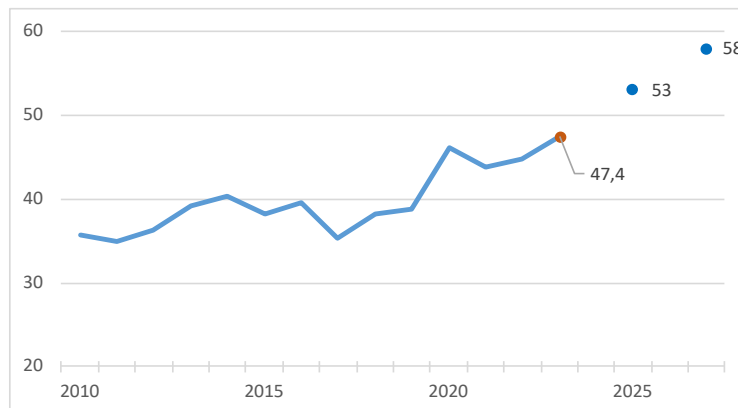
Gráfico 9. Proporción de enerxías renovables no consumo final bruto de enerxía. Anos 2010-2023 obxectivos a 2030. Galicia. Porcentaxe.
