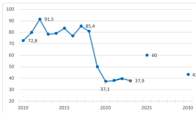
Gráfico 1. Redución das emisións de GEI. Galicia. Anos 2010-2023 e obxectivos a 2030.
